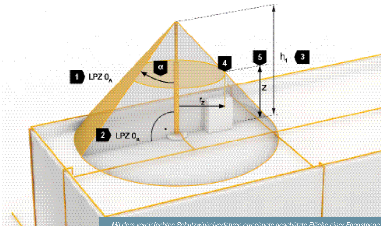
Mit dem vereinfachten Schutzwinkelverfahren errechnete geschützte Fläche einer Fangstange
